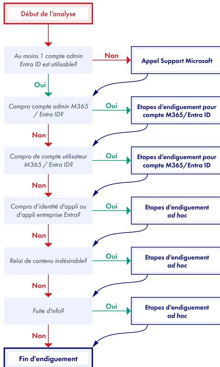
Figure 1 – Étapes de qualification et d'endiguement
