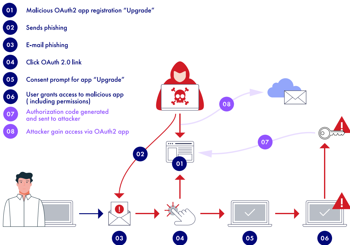
Figure 3 – Étapes de phishing
