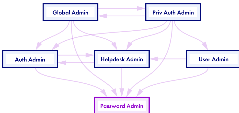
Figure 2 – Chemins de contrôle entre rôles Entra ID
